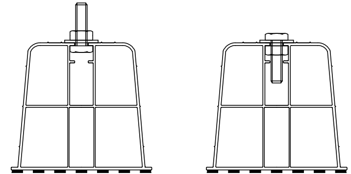
固定材図
