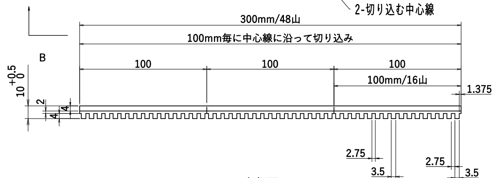
B矢视图
