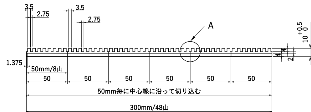
A矢视图
